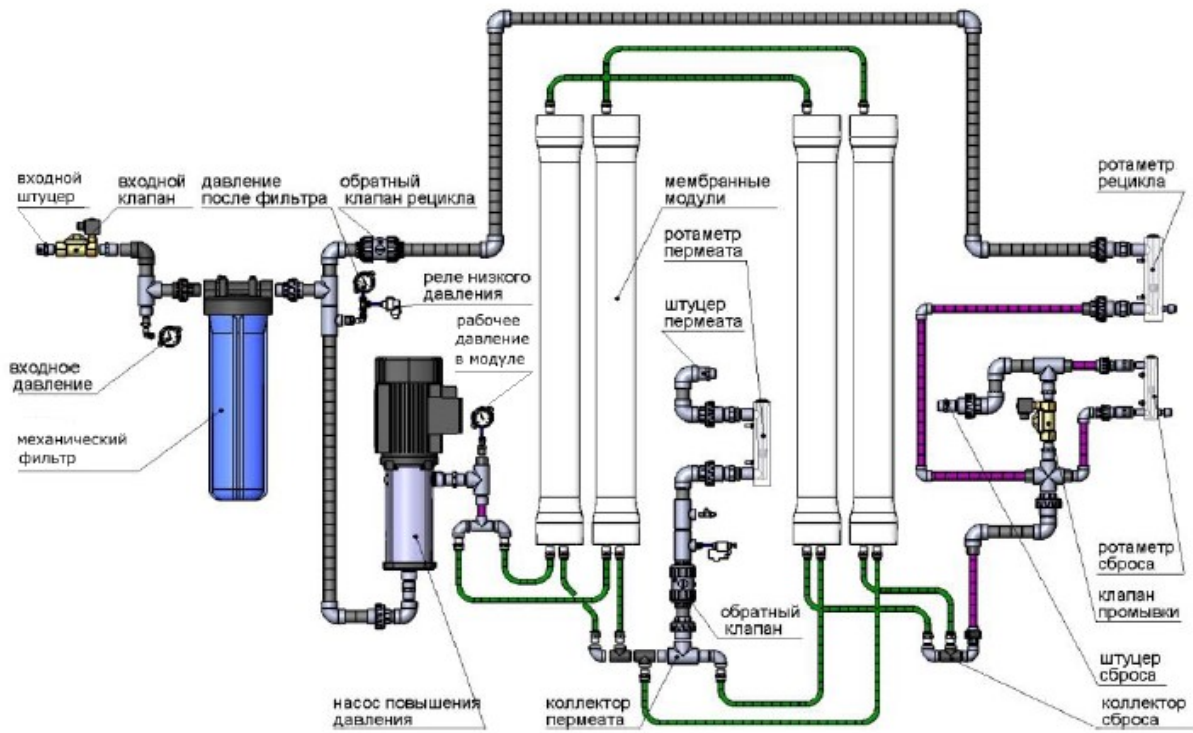
Рисунок 3. Схема системы обратного осмоса MO24000
