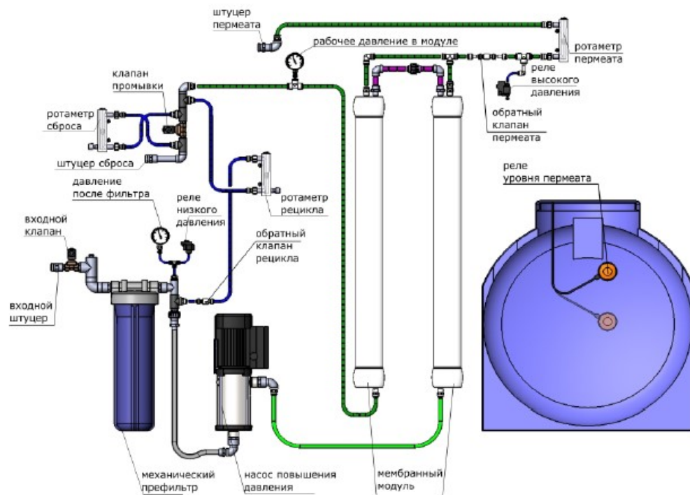
Рисунок 2. Схема системы обратного осмоса MO12000
