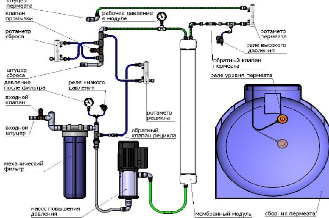
Рисунок 1. Схема системы обратного осмоса MO6000
