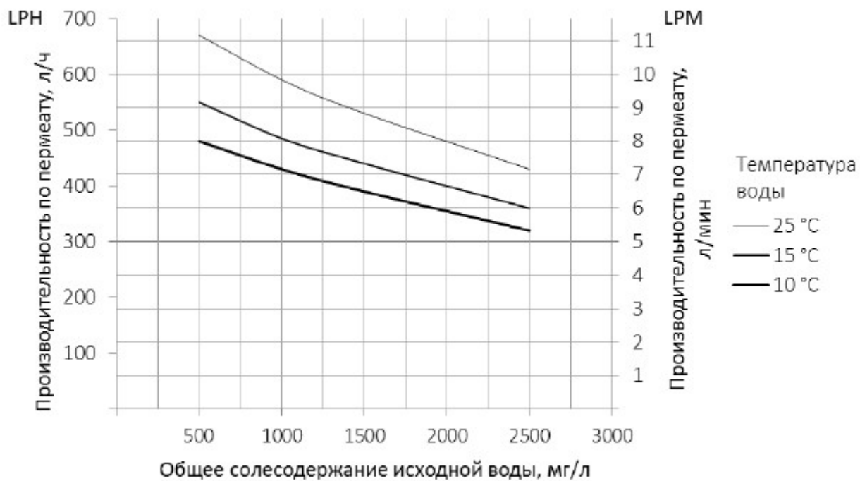
График 2. Зависимость производительности обратного осмоса MO12000 от общего солесодержания исходной воды
