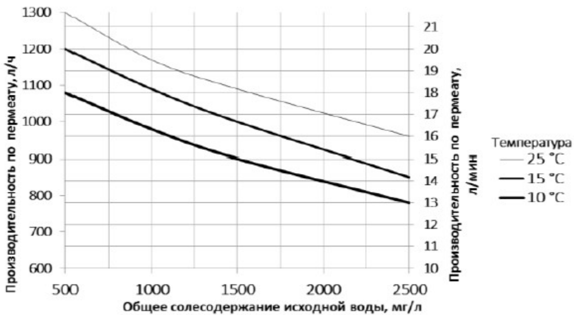
График 3. Зависимость производительности обратного осмоса MO24000 от общего солесодержания исходной воды
