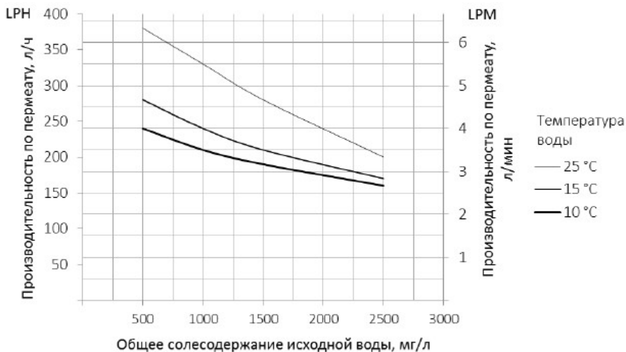
График 1. Зависимость производительности обратного осмоса MO6000 от общего солесодержания исходной воды
